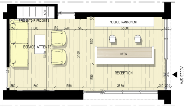
Plan d'aménagement
